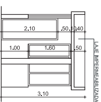
09 — Planta baixa - Guarita Esc.: 1/100
