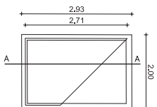
07 — Planta baixa - Guarita Esc.: 1/100
