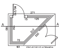
06 — Planta baixa - Garantia Esc.: 1/100
