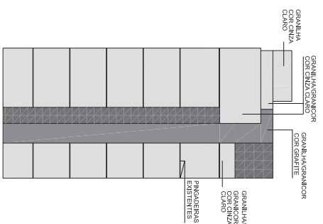
04 FACHADA AV. TOCANTINS Esc.: 1/200
