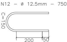
DETALHE DO CHUMBADO
