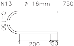
DETALHE DO CHUMBADO
