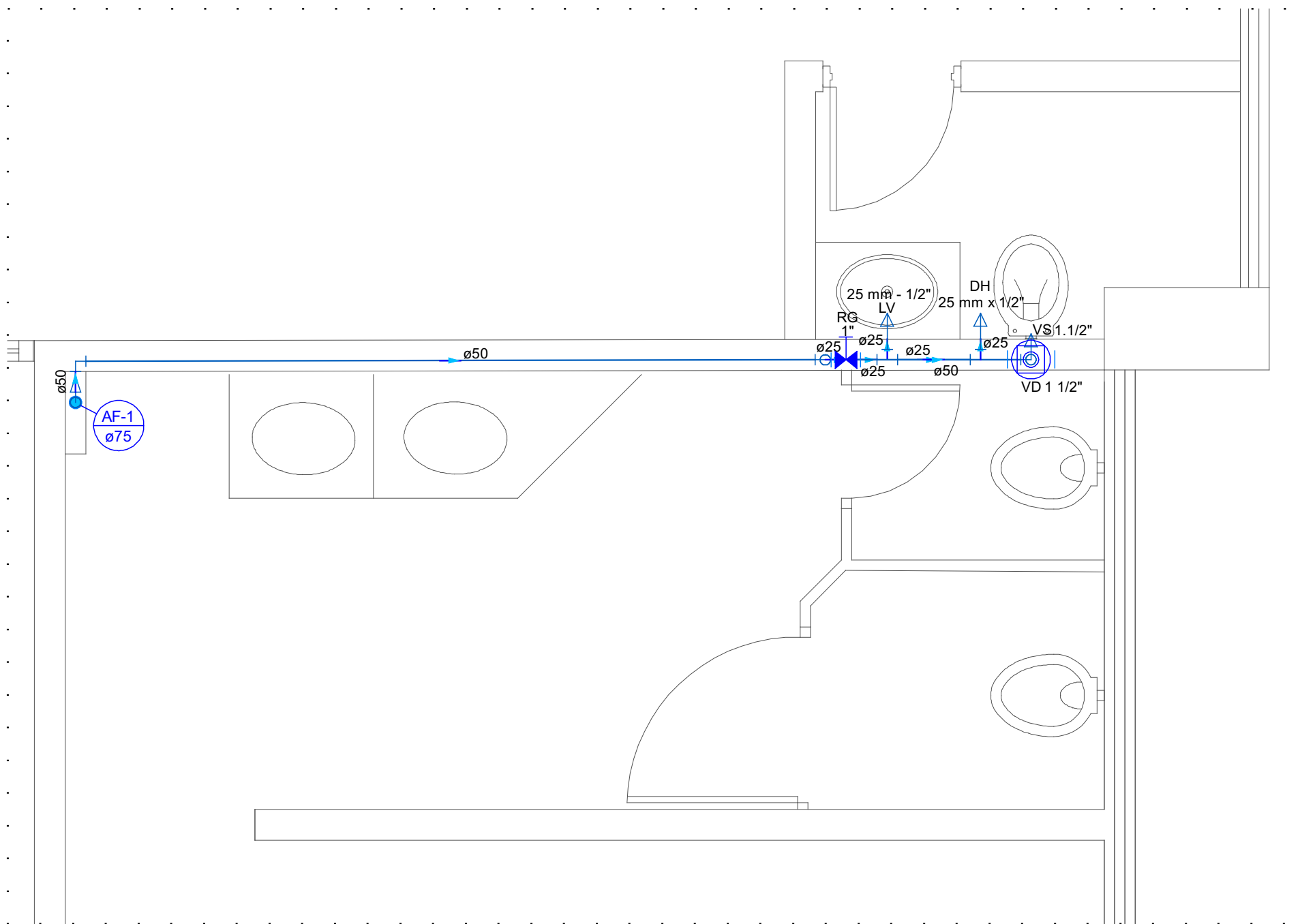
Detalhe HID-2 Escala 1:25
