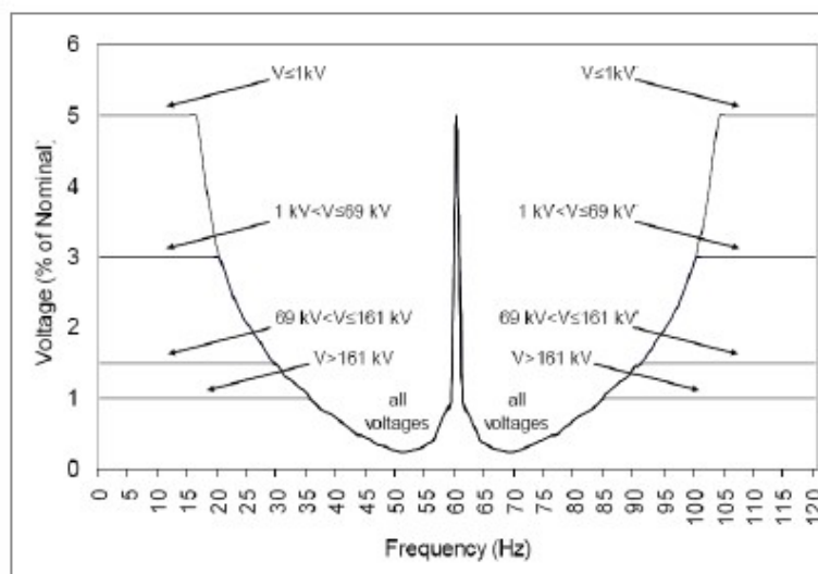
Figura 1: Limites para harmônicas de tensão
