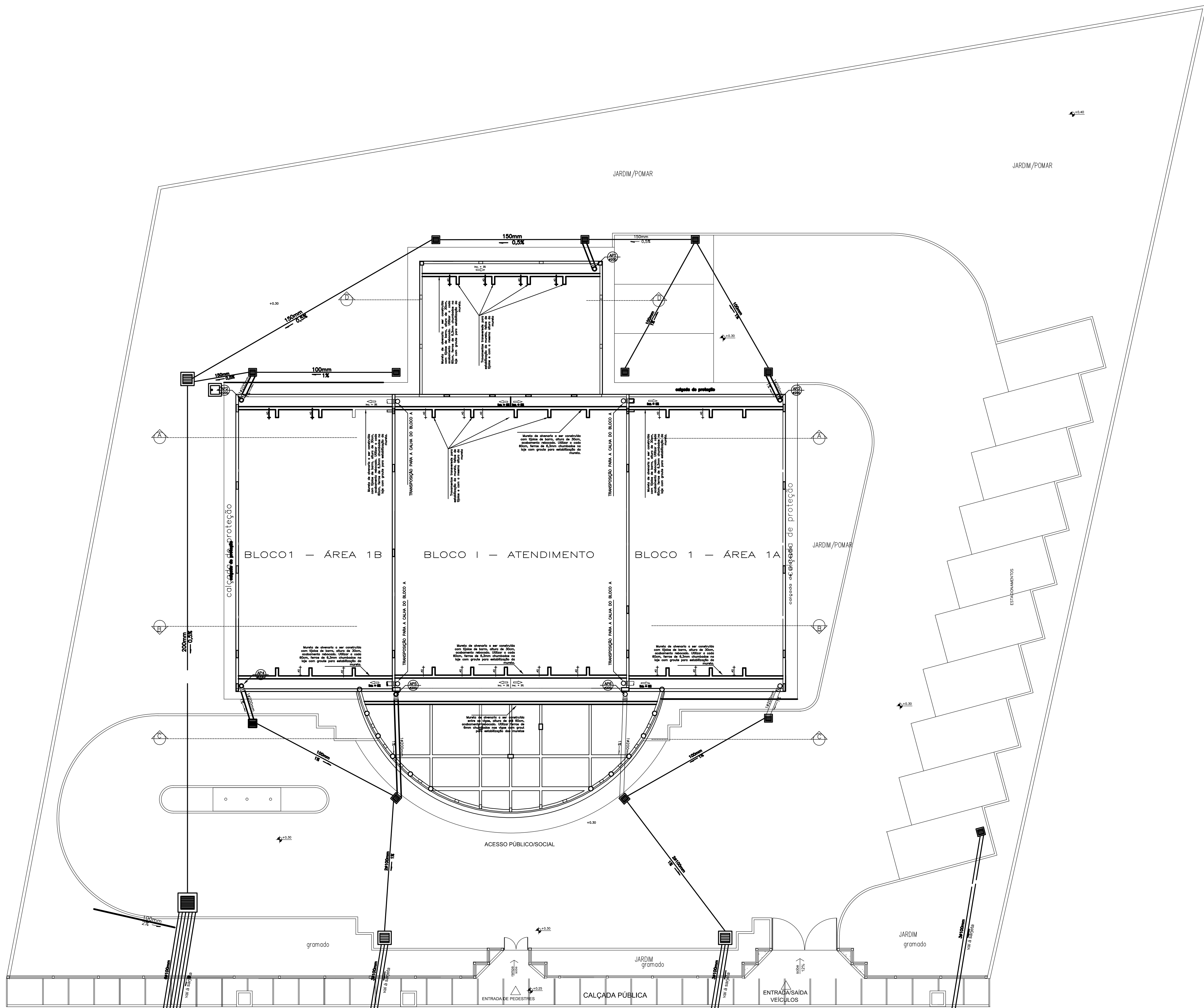
IMPLANTAÇÃO escala 1:100
