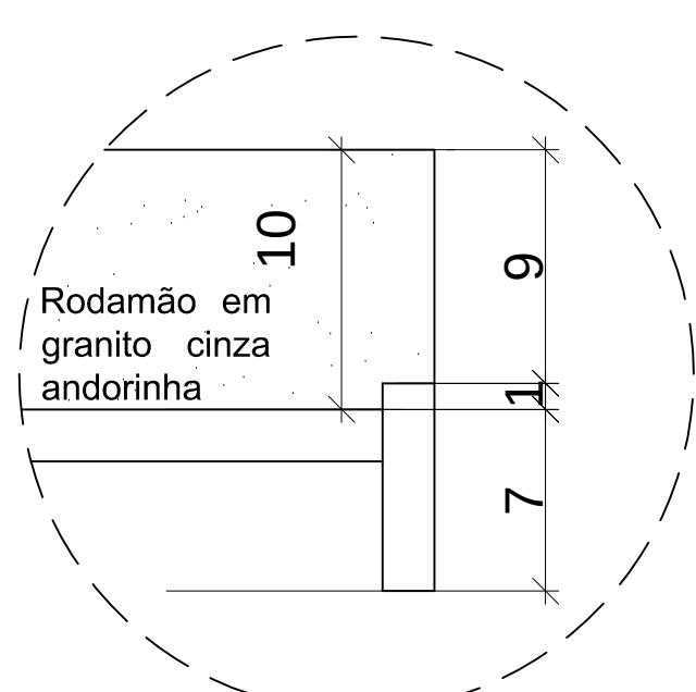
DETALHE GRANITO BANCADA 02 SEM ESCALA
