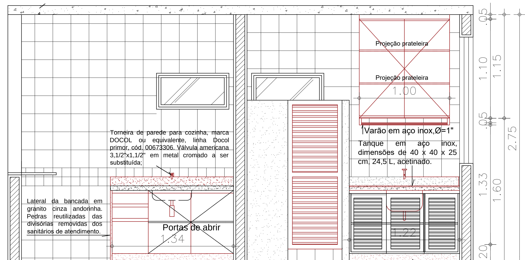
COPA - CORTE HH Esc.: 1/20
