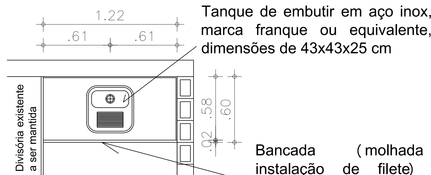
PLANTA BAIXA - BANCADA 2 Esc.: 1/20
