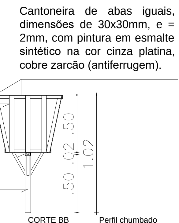
DETALHES LIXEIRA ESC.:1/20
