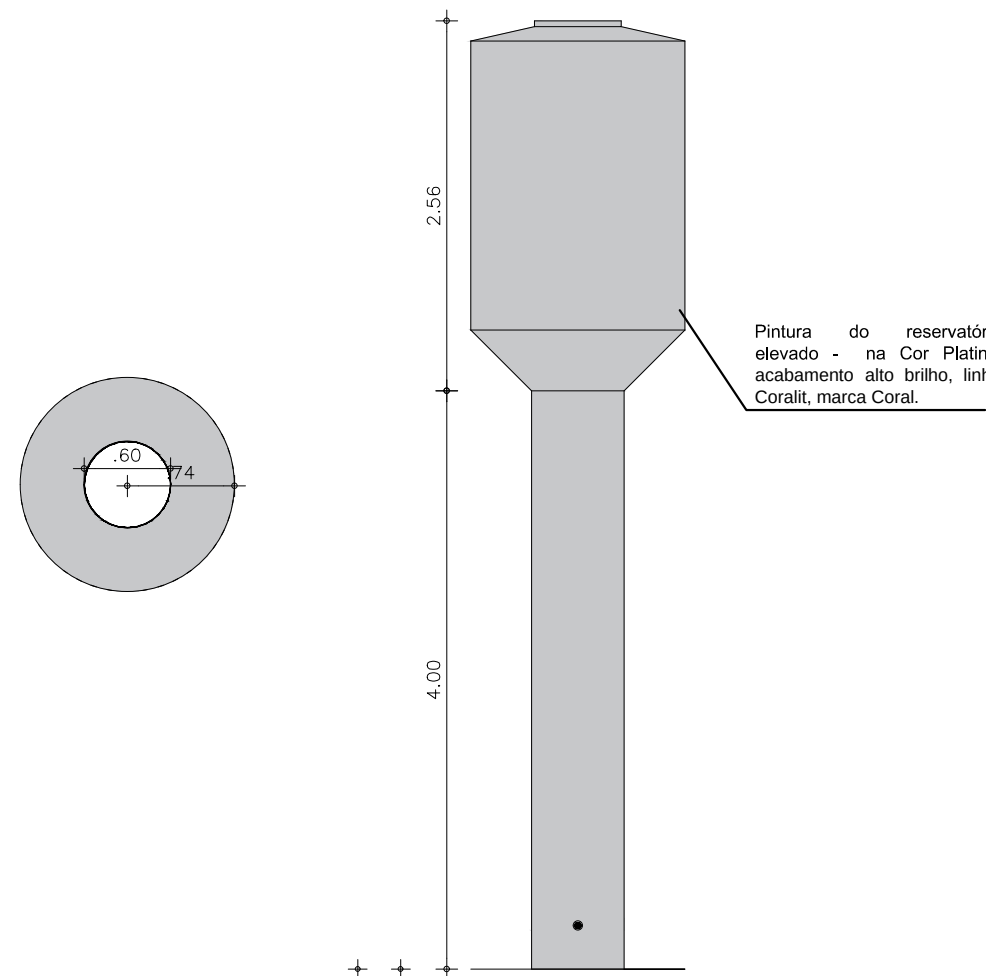
VISTA - RESERVATÓRIO ESC.: 1/50
