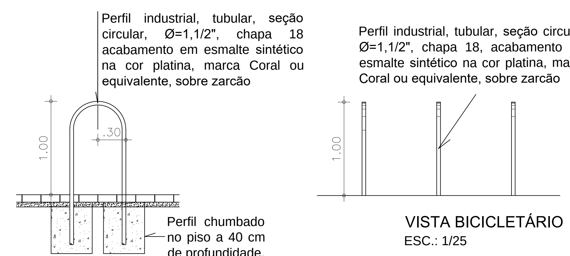
CORTE - BICICLETÁRIO ESC.: 1/25
