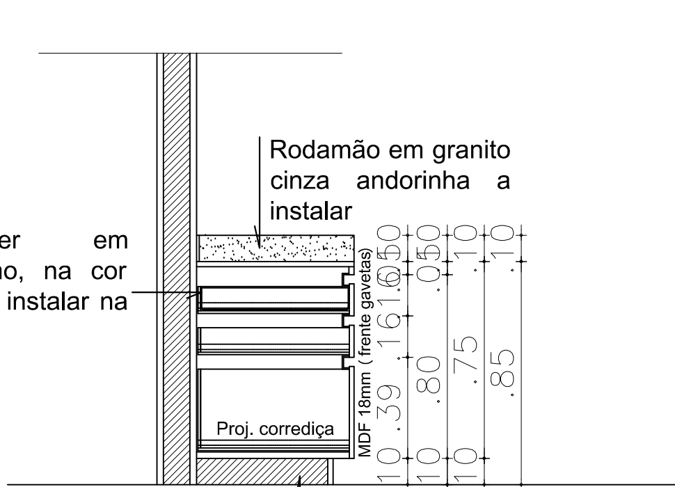
CORTE J Esc.: 1/20
