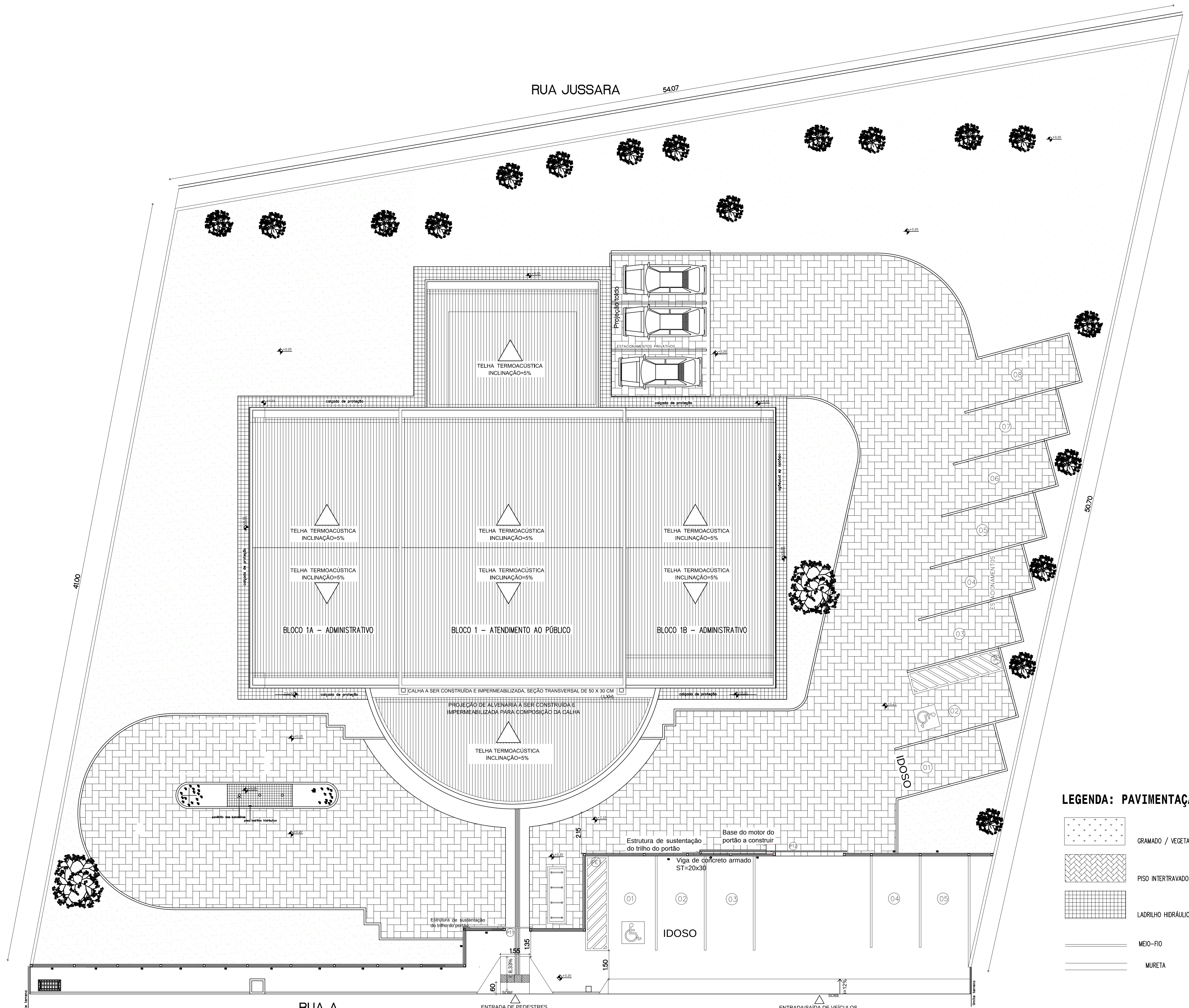
IMPLANTAÇÃO E COBERTURA - FINAL Esc.: 1/100
