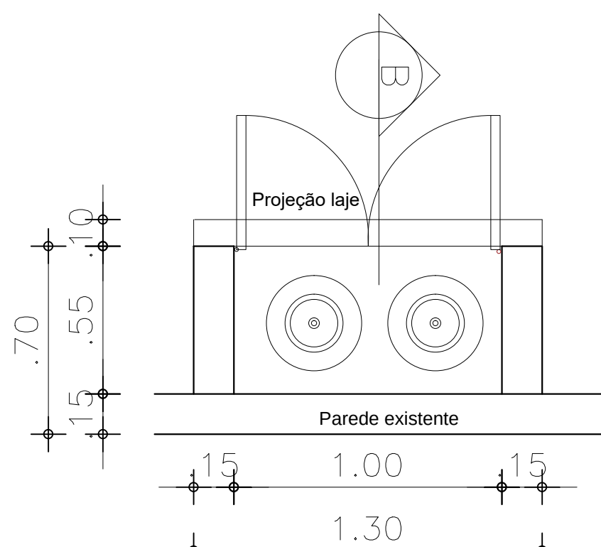
PLANTA BAIXA Esc.: 1/20
