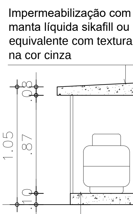
CORTE B Esc.: 1/20
