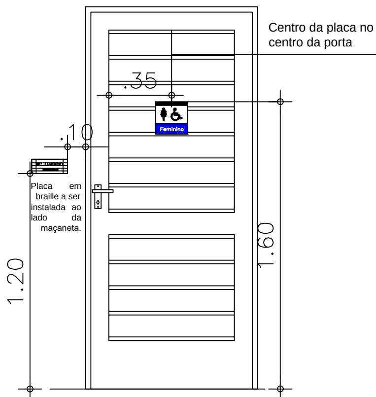
Vista 01 - Instalação de placas nas portas e paredes ESC. 1/20
