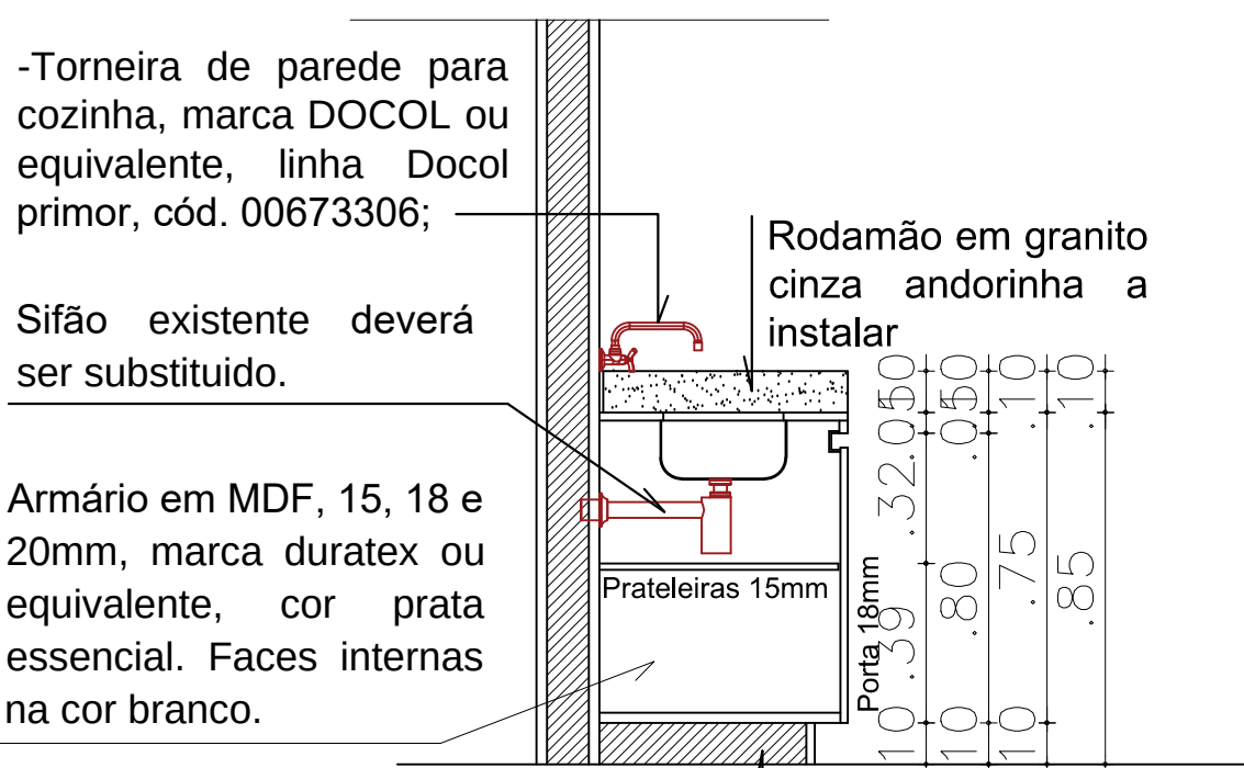
CORTE I Esc.: 1/20
