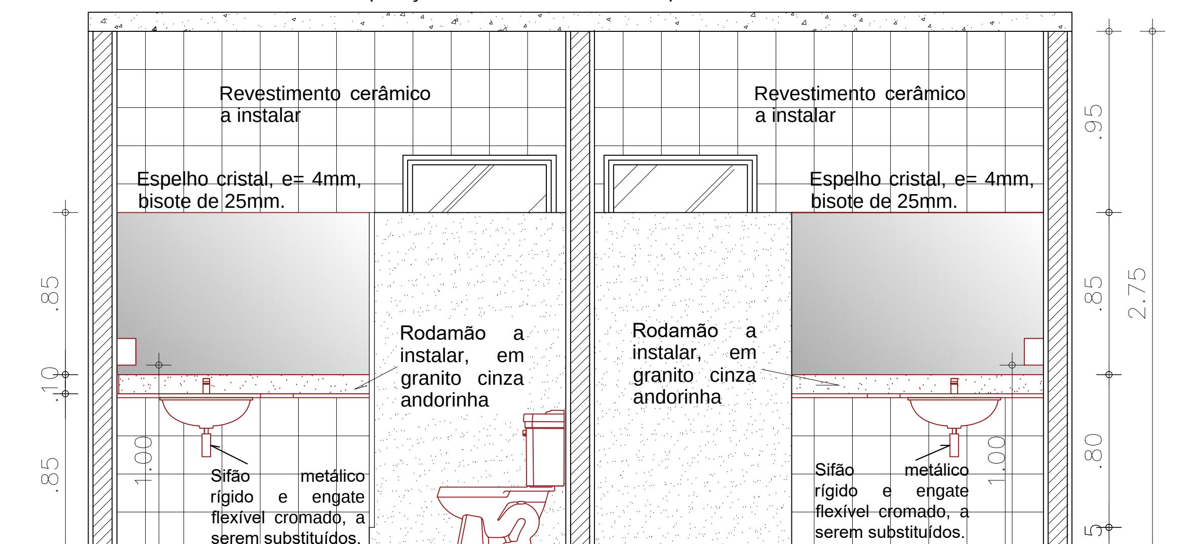
SANIT. FEMININO - CORTE LL Esc.: 1/20
