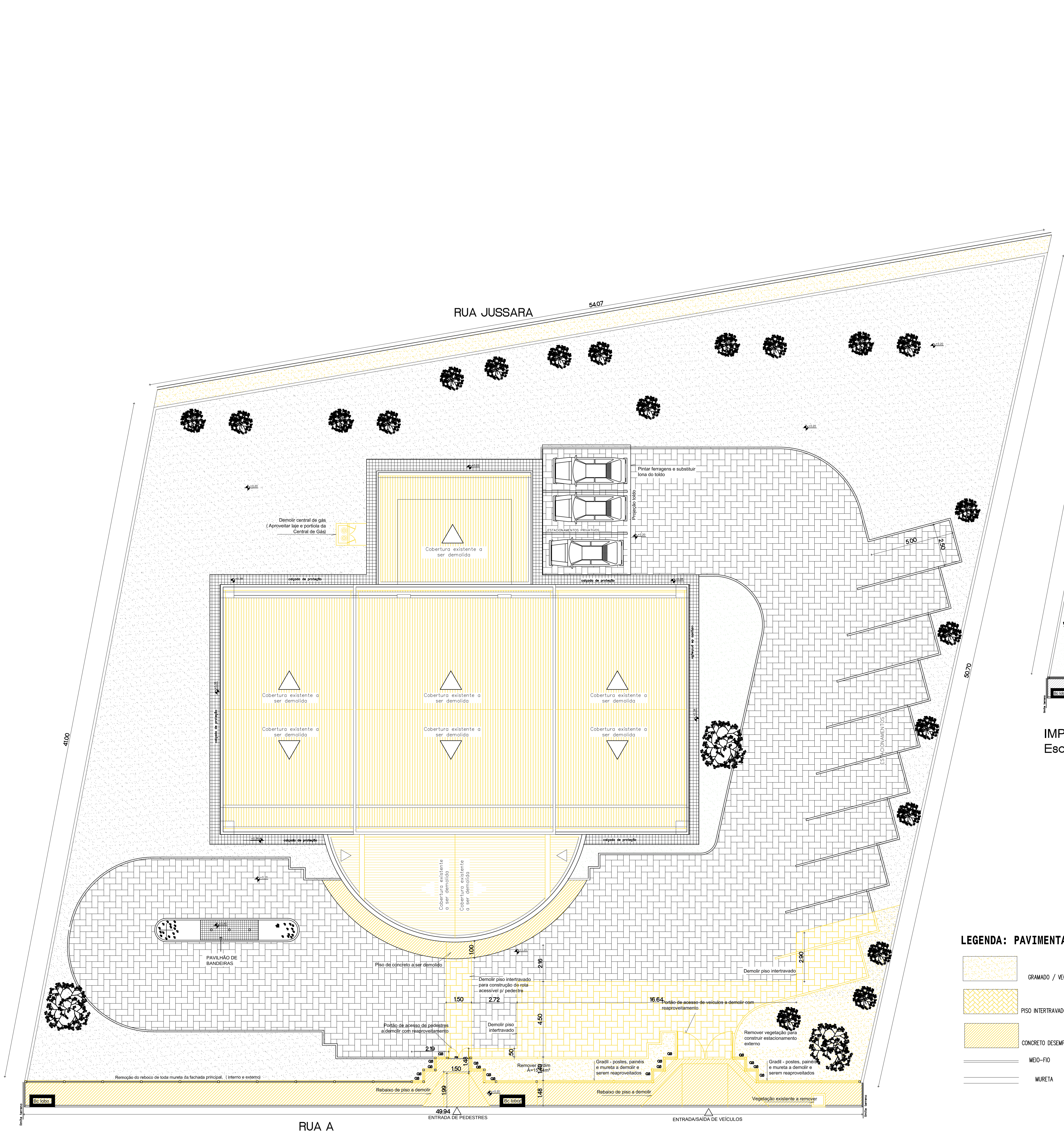
IMPLANTAÇÃO E COBERTURA - DEMOLIR Esc: 1/100
