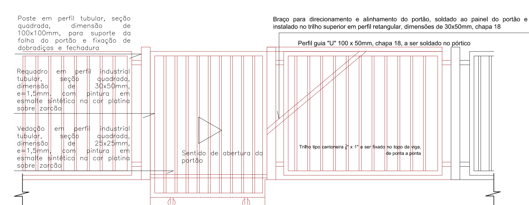
VISTA PORTÃO DE PEDESTRES-PT1 Esc.: 1/25
